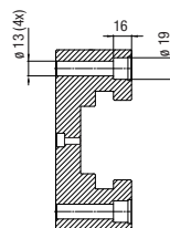
SEZIONE B-B
