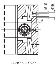
SEZIONE C-C
